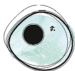
Нормална клетка
